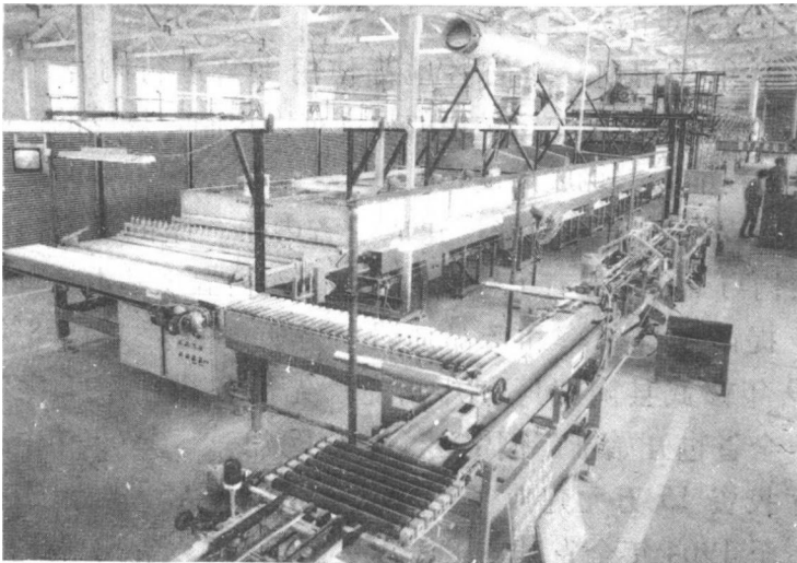
照 1—2—2 新美陶瓷有限公司引进意大利的全自动辊道窑
