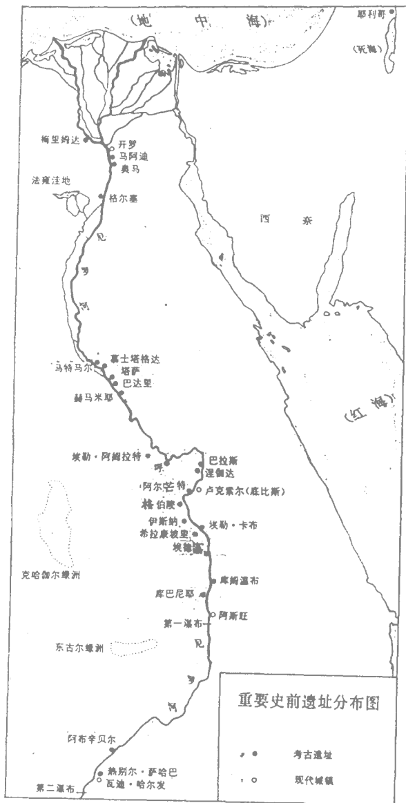
重要史前遗址分布图
