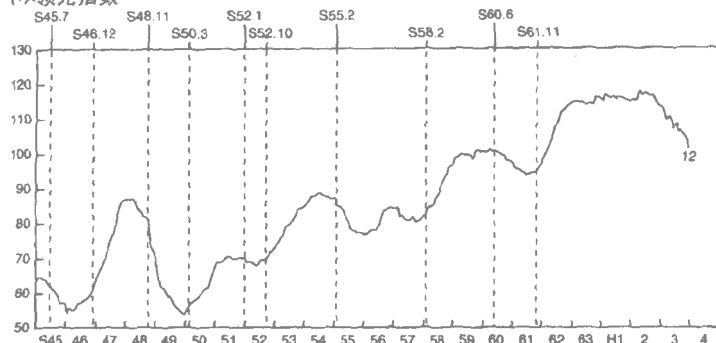
(2) 同步指数
