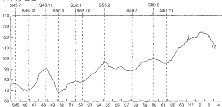
(3) 滞后指数
