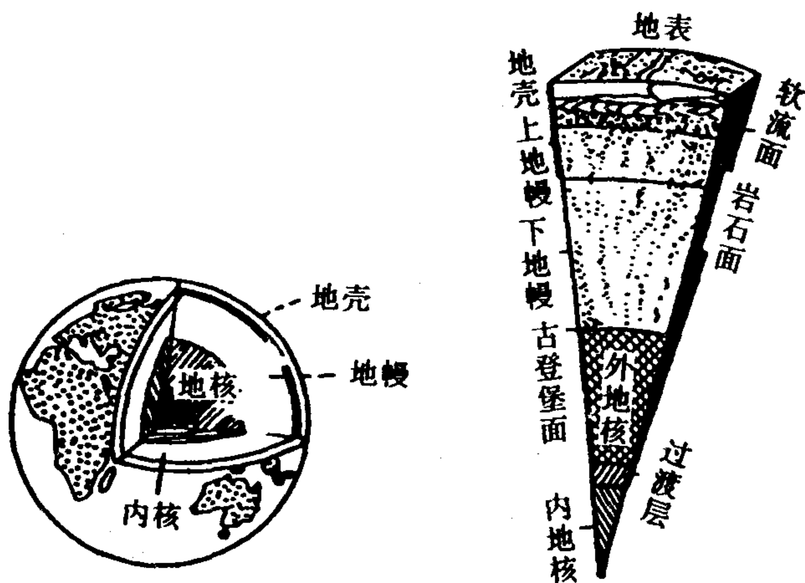
A. 地球内部的圈层结构
