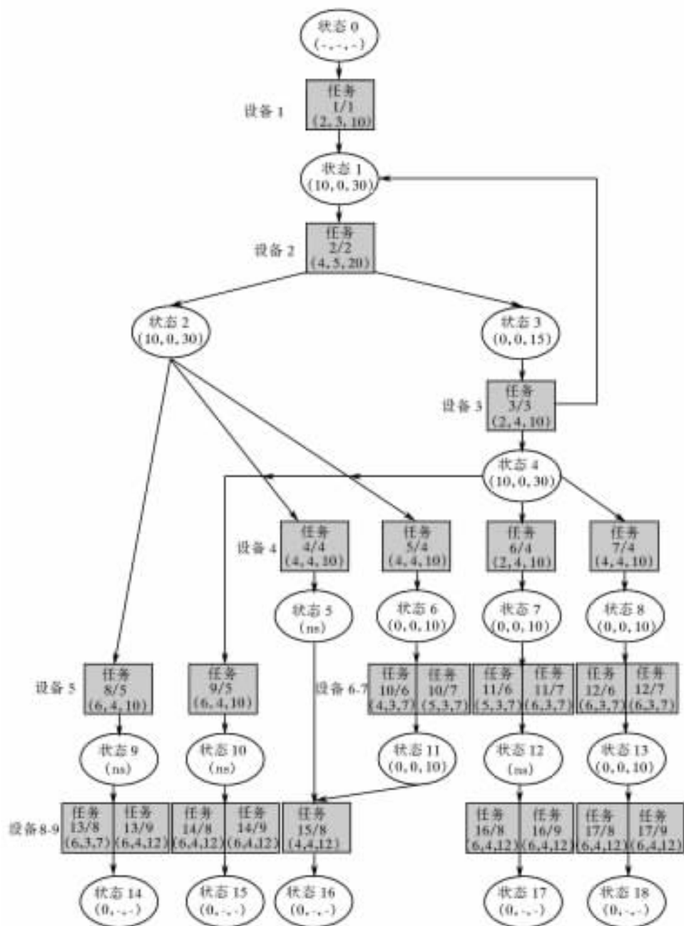
图 员 资源分配问题典型案例的状态任务网络图
