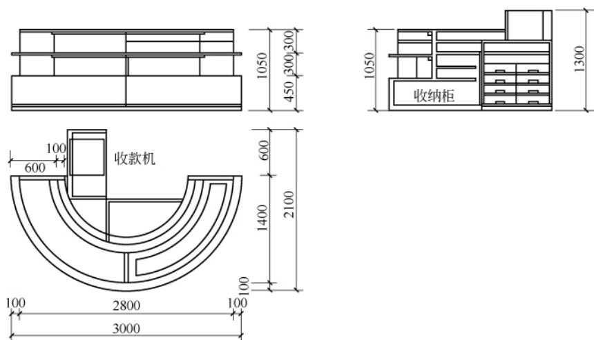
图 3-3-32 半圆形收银台三视图
