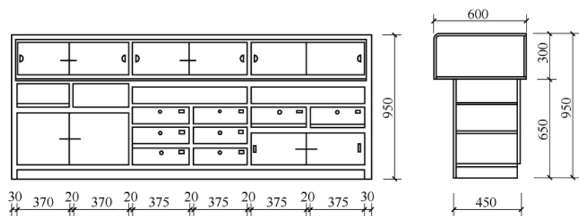
图 3-3-31 长方形陈列柜三视图
