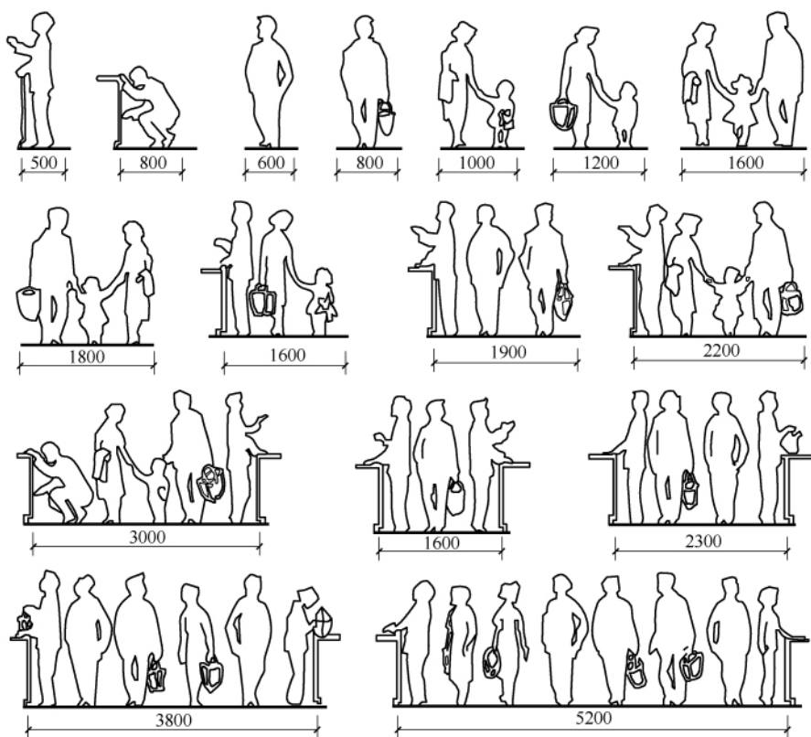
图 3-3-2 商场中的人体活动尺寸
