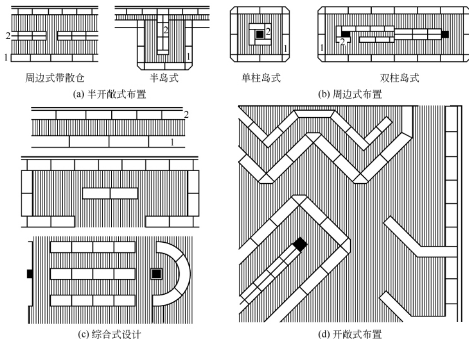
图 3-3-1 商场的平面布置 1—柜台; 2—货架
