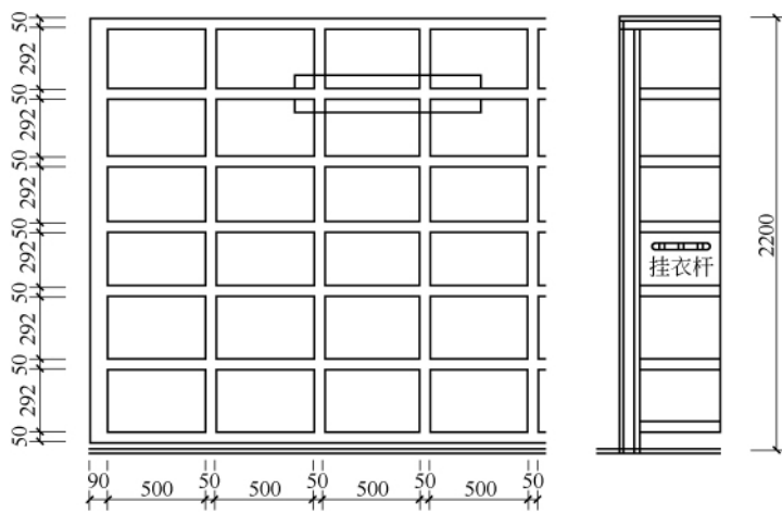
图 3-3-30 陈列架三视图
