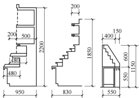
图 3-3-33 阶梯式陈列柜剖面
