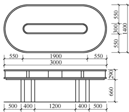
图 3-3-34 椭圆形陈列柜三视图
