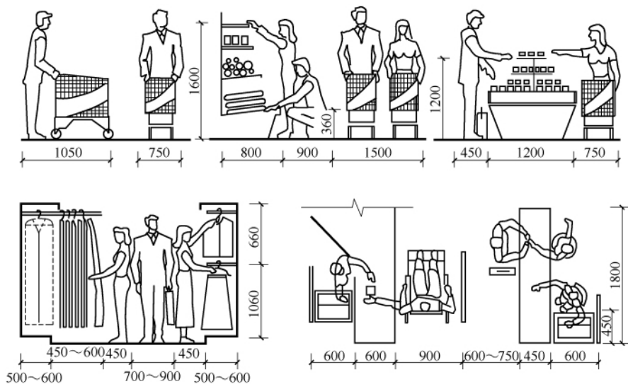
图 3-3-3 商场家具与人体尺寸
