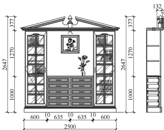
(b) 多功能书柜三视图
