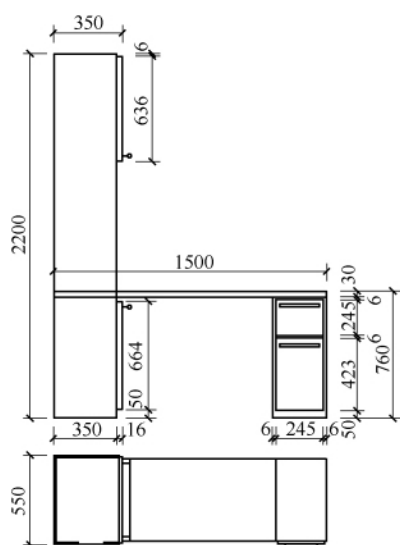
图 2-5-18 钢木框架式书房家具
