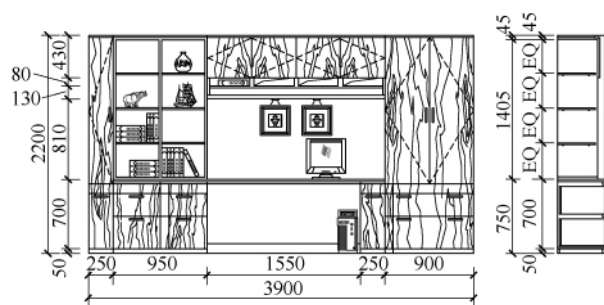
(b) 多功能书柜三视图
