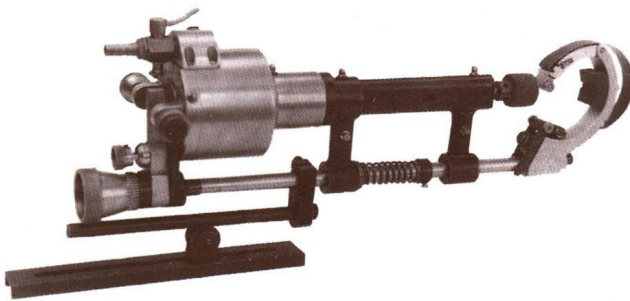
1965年革新自制的手动式曲轴光磨机
