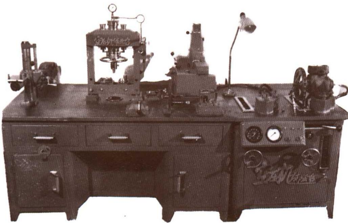
1976年革新自制的空气压缩机作业试验台
