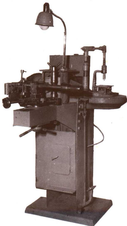
1965年革新自制的制动蹄片光磨机
