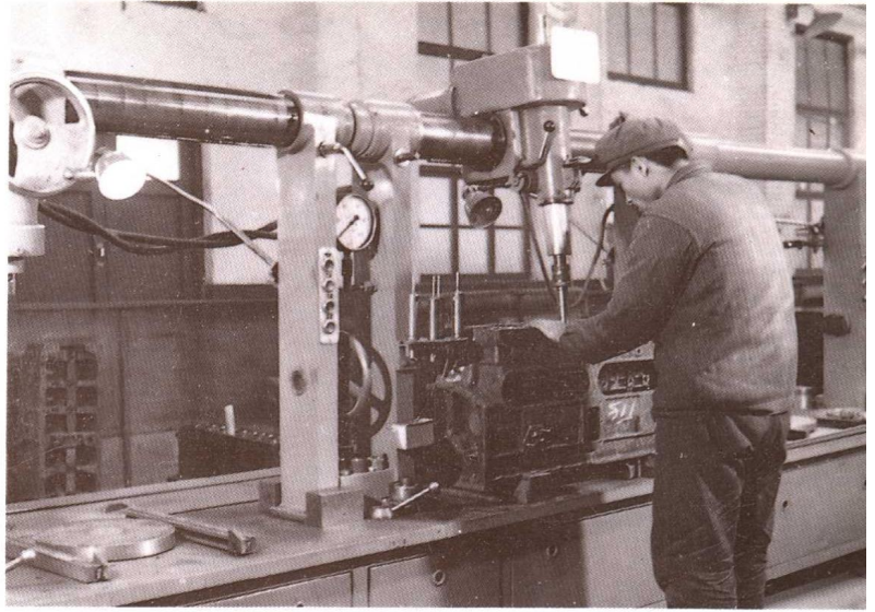
镗缸前缸体加工作业台
