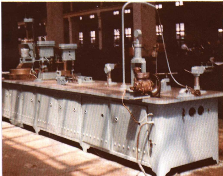
张家口汽车修理厂革新制造的气泵作业台
