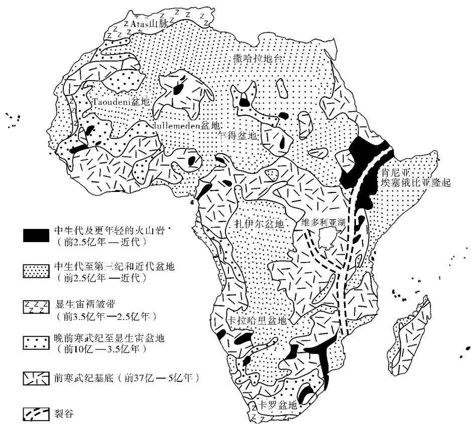
图 2-1 非洲地质纲要图（显示基底露头 and 盆地） (资料来源：地质部地质研究所编，地质出版社，1980 年)
