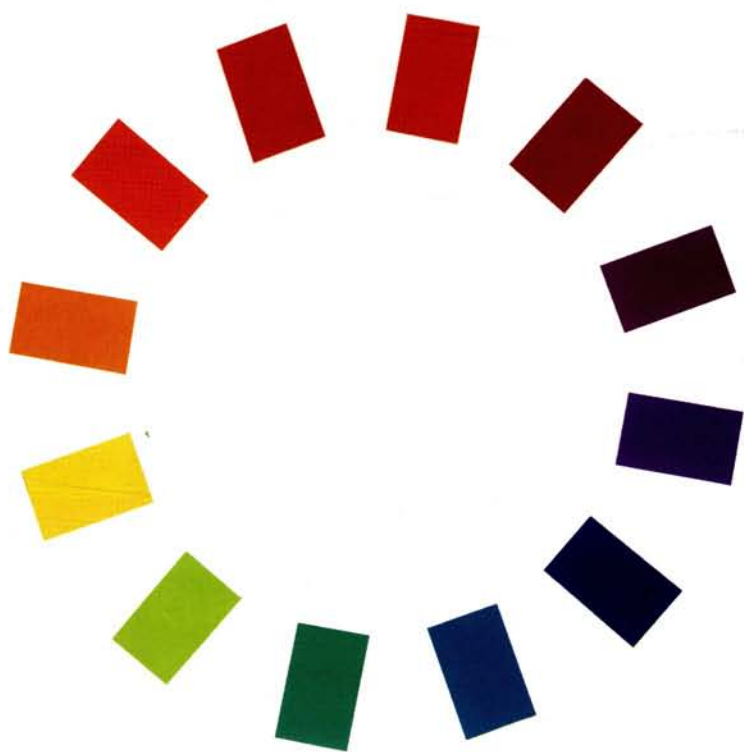
图1-6 12色相环
