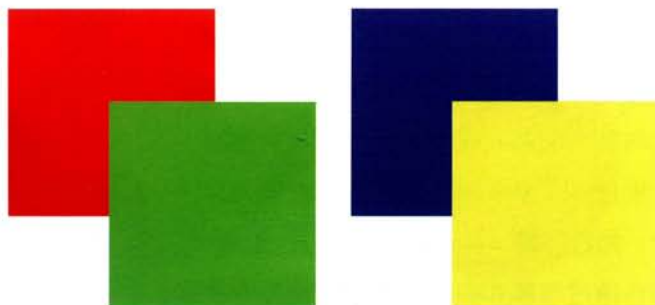
图1-8 补色
