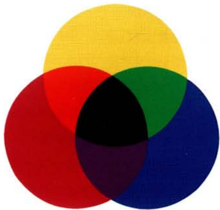
图 1-4 减色混合
