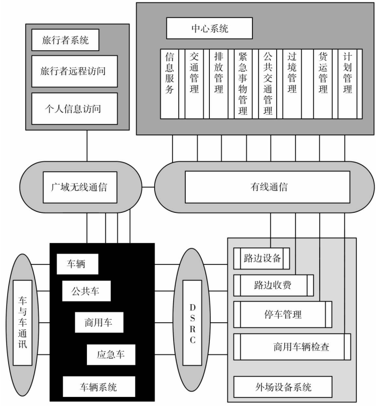
图 美国的基本框架示意图
