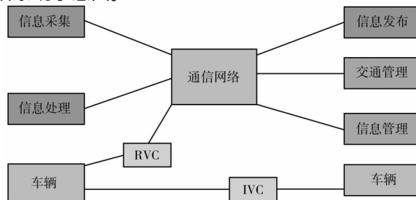
图 1-1 智能交通通信系统示意图
