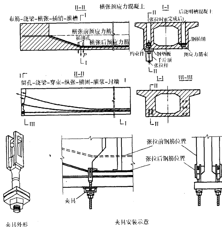
图 1-1-3 横张预应力示意图
