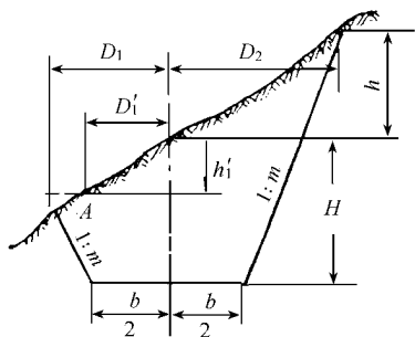
图 1.2.3 坡地上放边桩示意图
