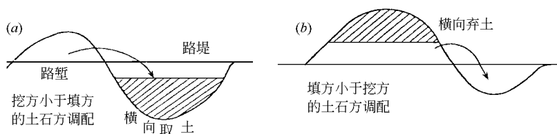
图 1.3.4 土石方调配示意图
