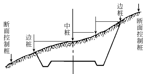
图 1.2.1 路基桩点布置图
