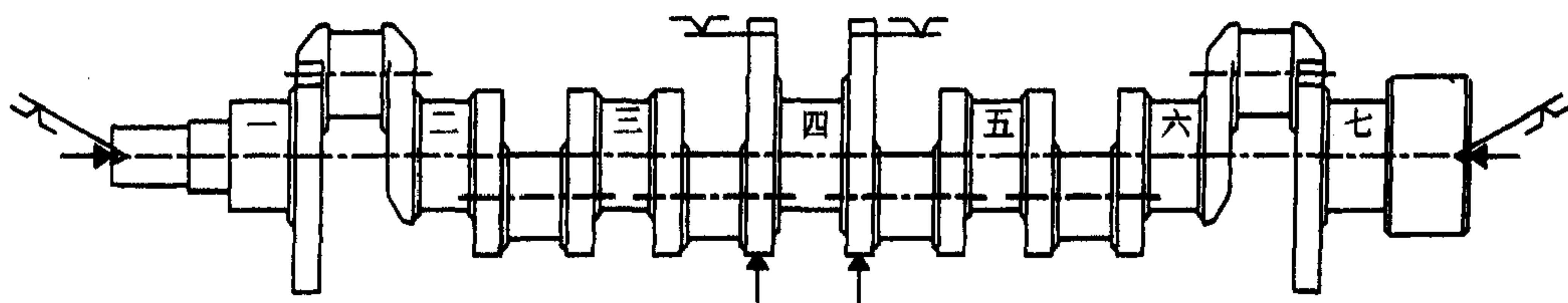
图 1-2 曲轴定位夹紧示意图
