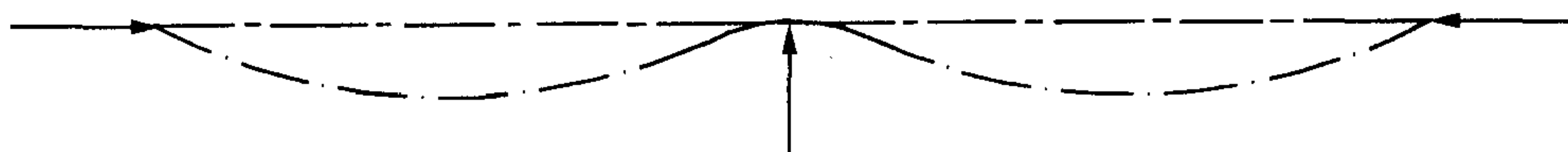
图 1-5 主轴颈轴线二次弯曲图
