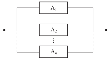
图1-7 并联系统
