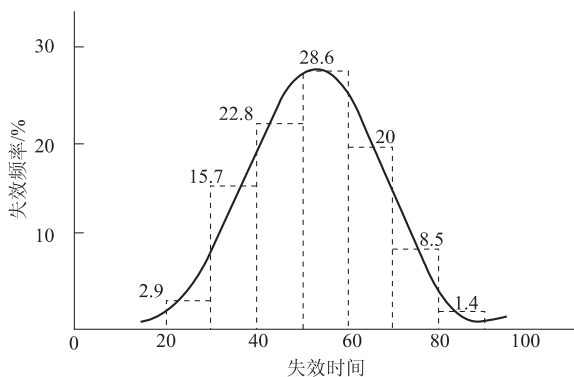
图 1-5 失效频率的直方图
