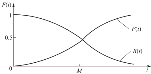
图 1-2 可靠度与不可靠度的关系曲线
