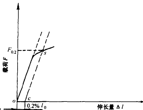
图 1-2 铸铁的力-伸长曲线
