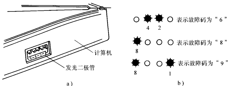
图 员原圆 采用四个 蕴纟显示故障码举例
