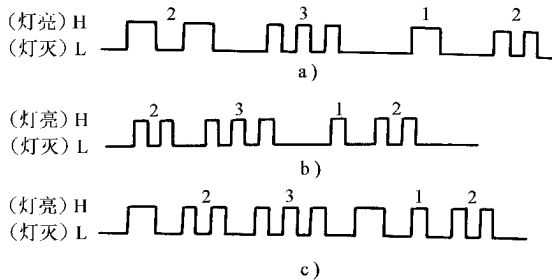
图 员原员 故障码“圆猿”和“猿圆”的显示方法
