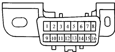
图圆 韵月阅原II 系统圆端子诊断插座的形状、位置和接头的布置
