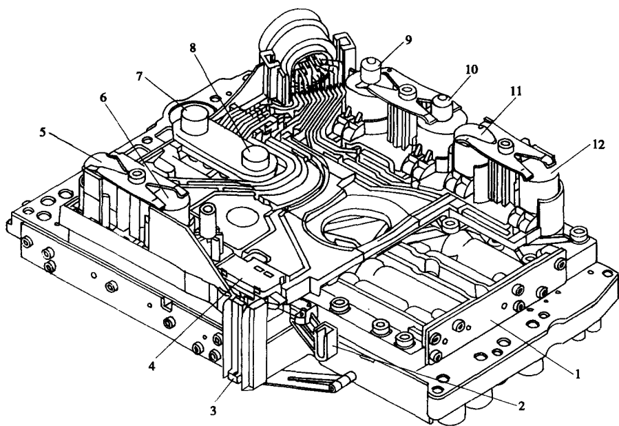
图 1-3 阀体部分的组成
