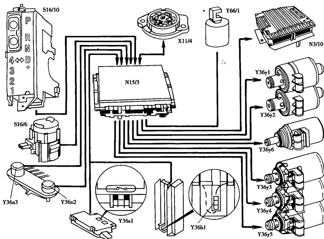
图 1-5 变速器电脑硬件信号的构成
