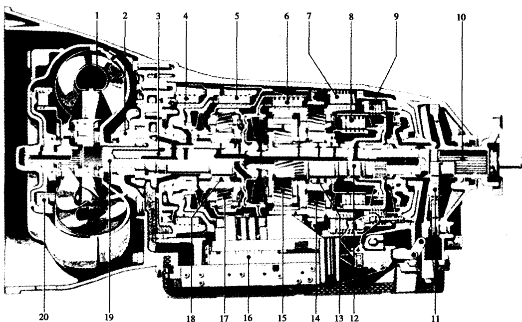
图 1-1 变速器构成元件及位置图
