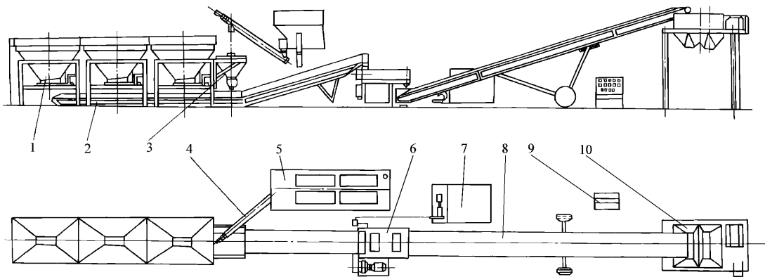
图 猿 稳定土厂拌设备
