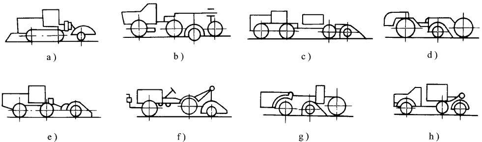
图 4-2 稳定土拌和机类型
