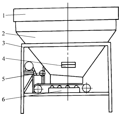
图 猿 配料机
