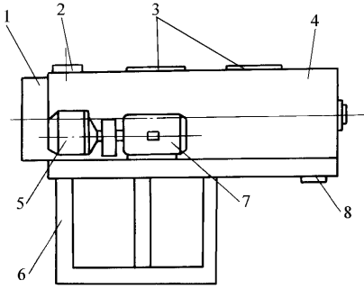
图 员缘 搅拌机
