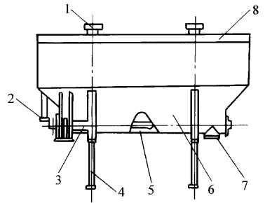
图 2 卧式存仓
