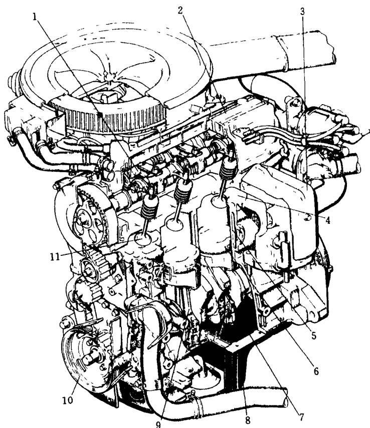
图 1-2 发动机的材料适用例
