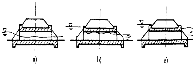
图 3 涵洞按水力性质分类
