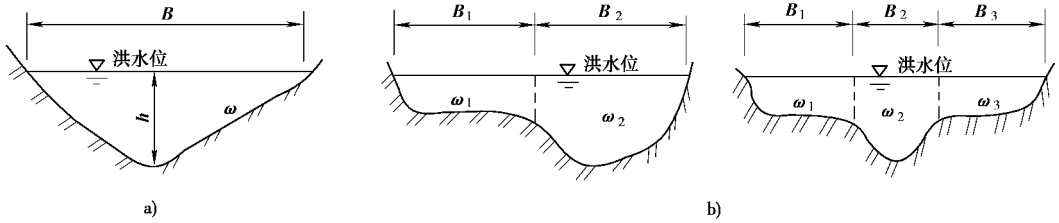
图 1-10 单式和复式横断面 单式断面 复式断面
