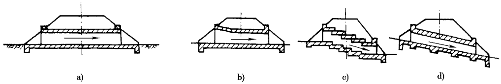
图 1-2-10 涵洞按洞身形式分类 a) 进口不抬高, 洞身平置式; b) 进口抬高, 洞身平置式; c) 进口抬高, 洞身斜置式; d) 进口抬高, 洞身斜置式
