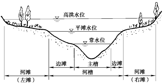
图 圆爱 摇河床横断面图
