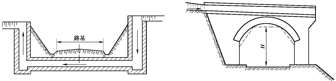
图 5-17 倒虹吸涵洞
