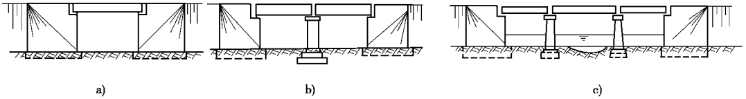
图 2 桥涵按孔数分类
