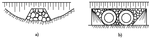
图 5-16 块石透水路堤
