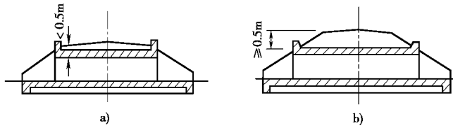
图 1 涵洞按填土高度分类
