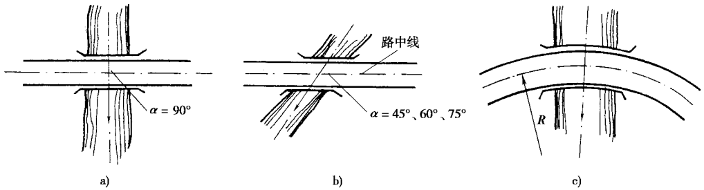
图 1-2-11 小桥涵按洞身平面布置分类 a) 正交桥(涵); b) 斜交桥(涵); c) 曲线桥(涵)
