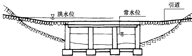
图 1-2 漫水桥
