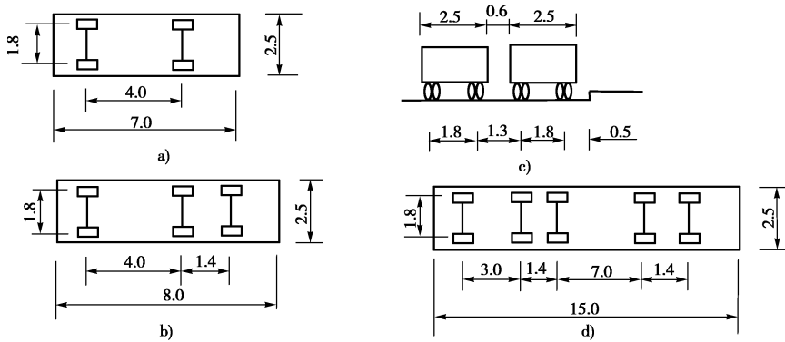
图 1-1 各种设计车辆平面尺寸和横向布置图(尺寸单位:米)
