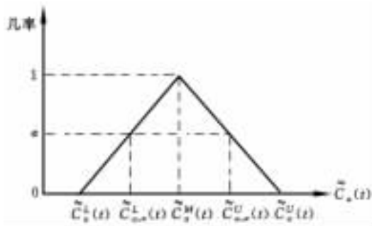
图 1-1 三角形几率分布
