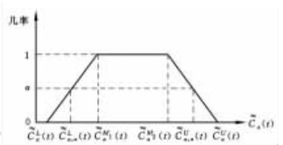
图 1-2 梯形几率分布
