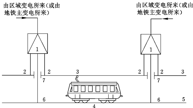
图 4-1 地铁供电系统示意图
