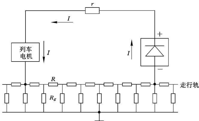
图 4-1-1 轨道—地的电阻分布网络
