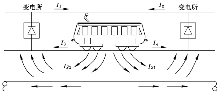
图 4-2 地铁杂散电流形成示意图
