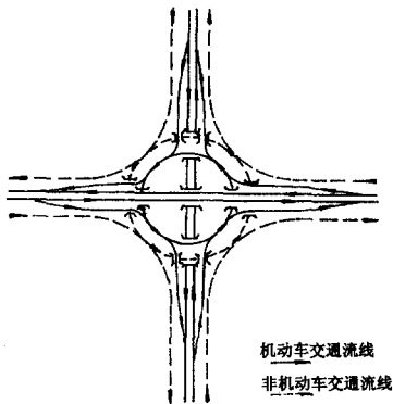
图 6.3.1-11 环形分行立体交叉(四层)
