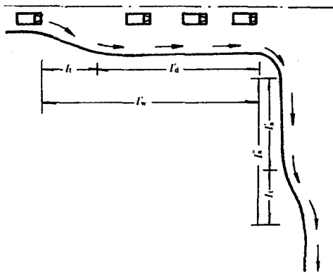
图 6.2.7 交叉口右转专用车道的设置
