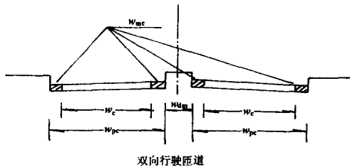
双向行驶匝道
