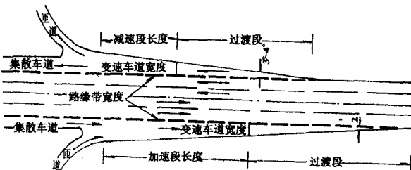
图6.3.10-1 直接式变速车道
