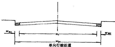
单向行驶匝道
