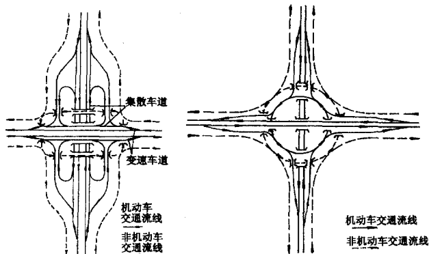
图 6.3.1-10 长条苜蓿叶形分行立体交叉(三层)
