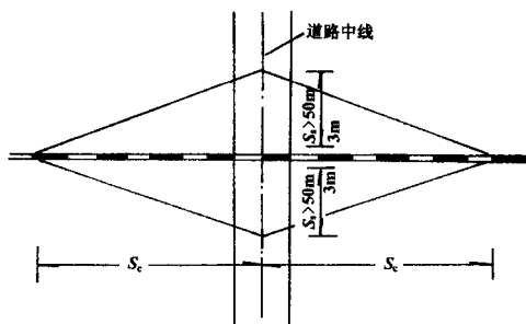
图 7.2.7 道口视距三角形
