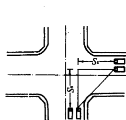
图 6.2.5-1 十字形交叉口 视距三角形
