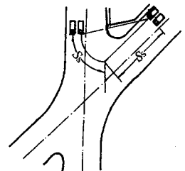
图 6.2.5-2 X形交叉口 视距三角形
