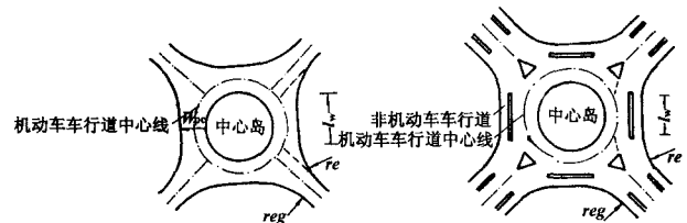
图 6.2.11 环形交叉口
