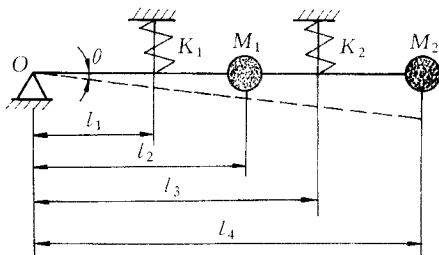
图 1.2 例 1.2 的系统
