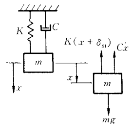
图 员源 员 粘性阻尼振动系统
