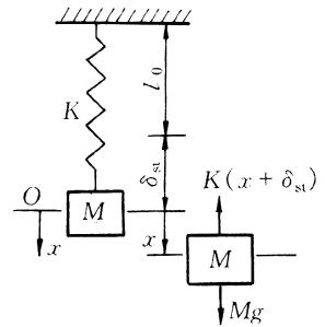
图 1-1 质量-弹簧系统
