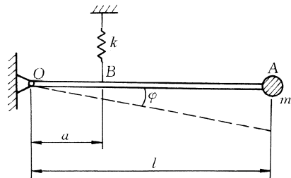
图 1.1 例 1.1 的简图
