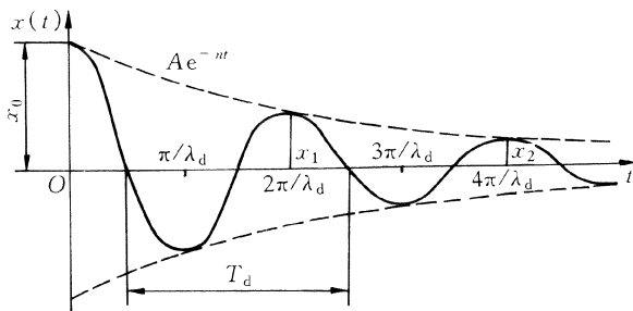
图 15-15 有阻尼自由振动(指数衰减振动)
