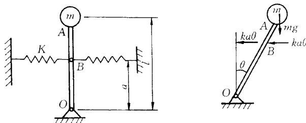
图 1-1-1 倒置摆
