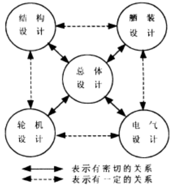
图 1.1.1 船舶设计关系框图
