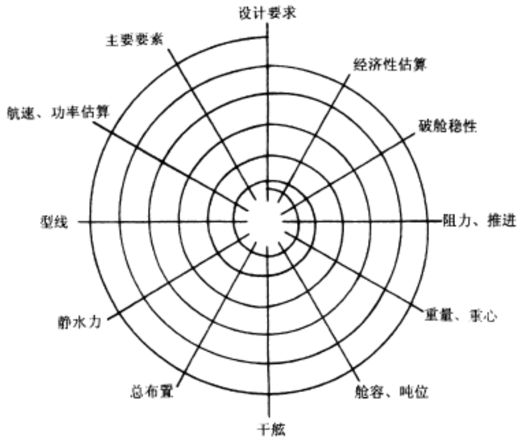
图 1.2.1 总体设计螺旋线
