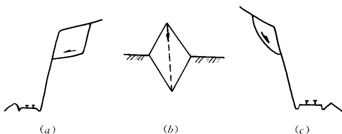
图 1-2 滑移—崩塌
