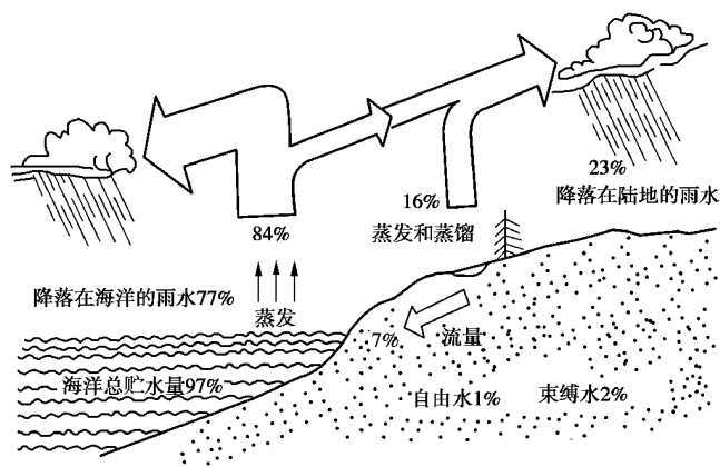
图 5-11 水的循环
