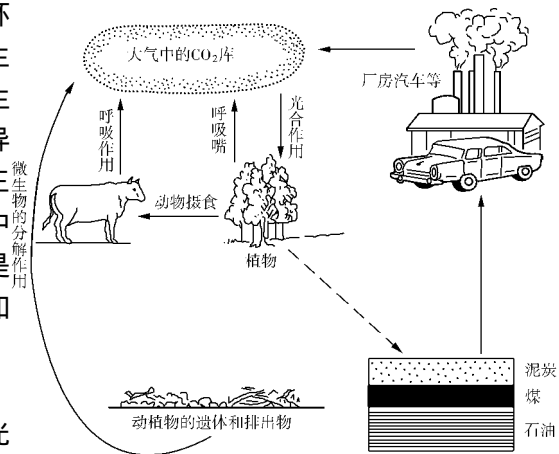
图 5-5-1 碳循环图
