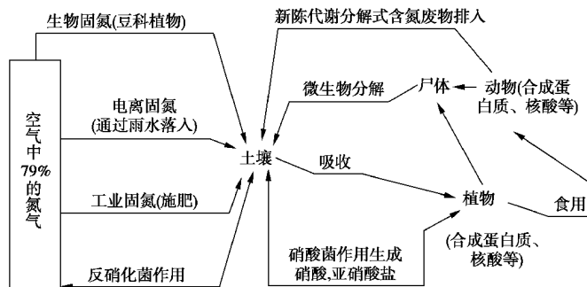
图 5-5-2 氮循环图
