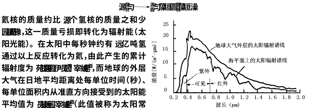
图 5-20 太阳发射光谱图
