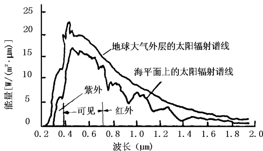
图 员 圆 太阳发射光谱图
