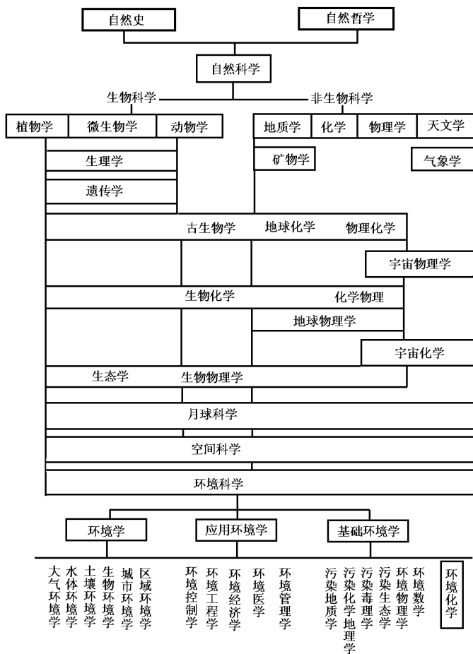
图 1-1 环境科学的学科组成及其在自然科学中的地位
