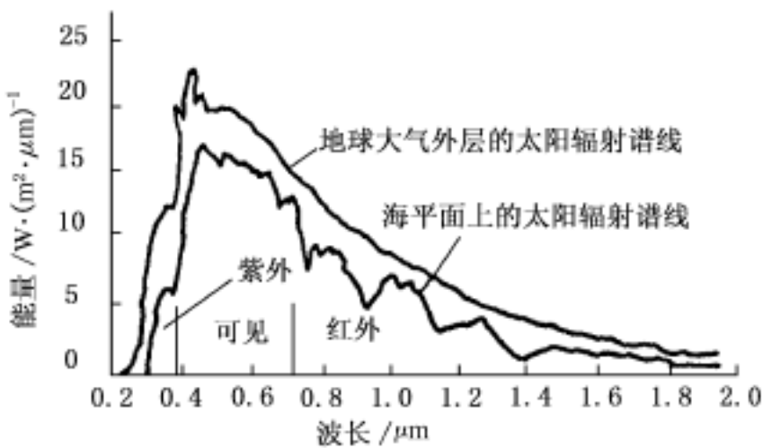
图 1-2 太阳发射光谱图
