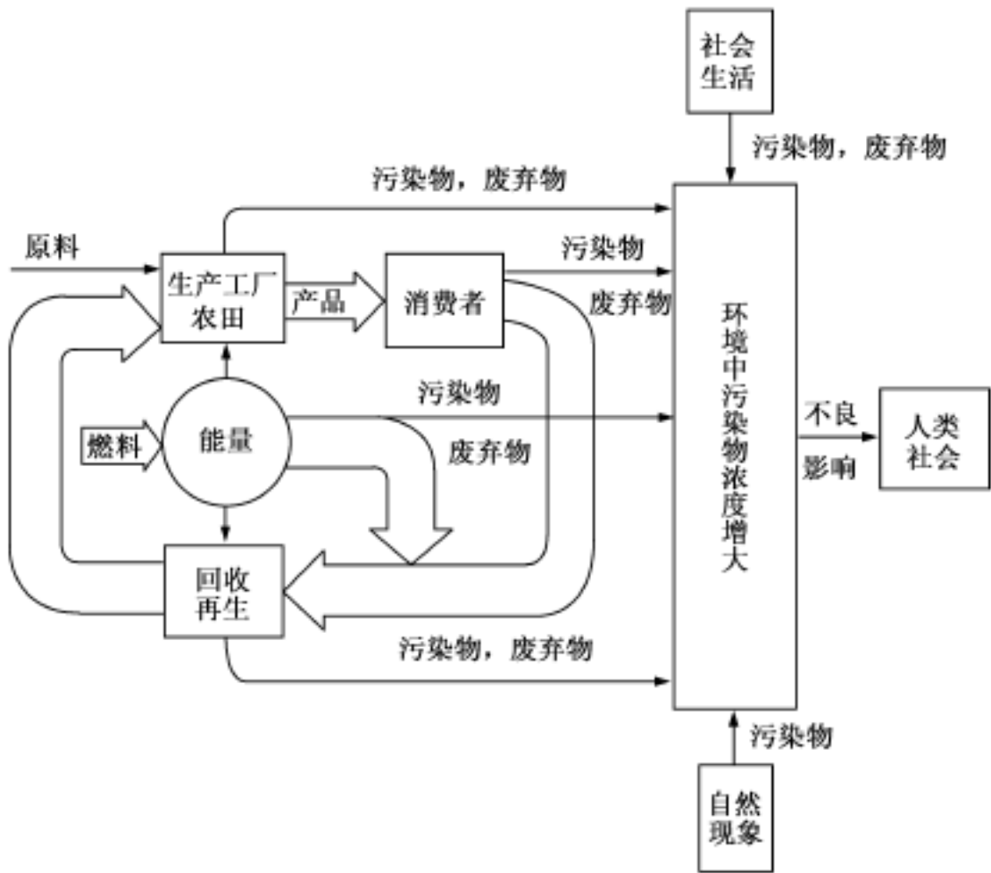
图 1-5 环境污染概念图
