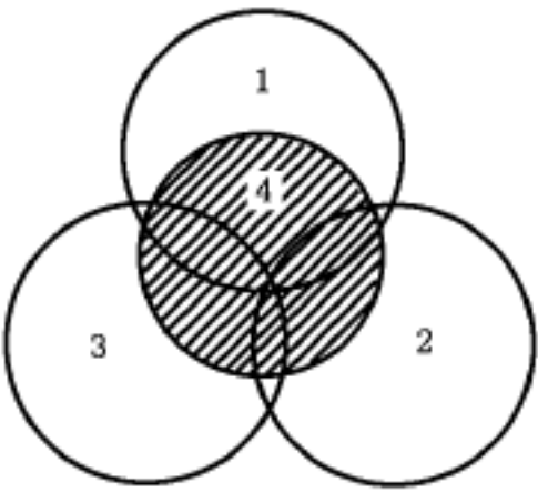
1. 大气圈 2. 水圈 3. 岩石圈 4. 生物圈
