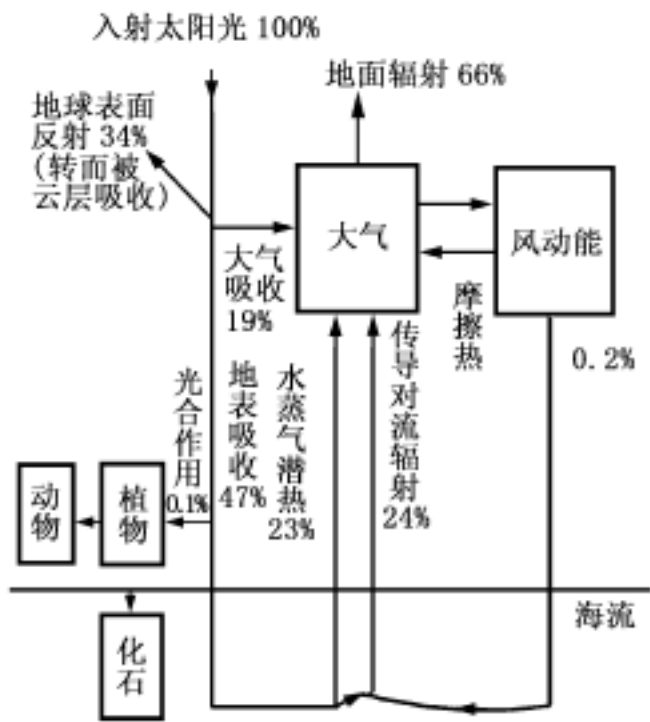
图 1-3 太阳能的流动
