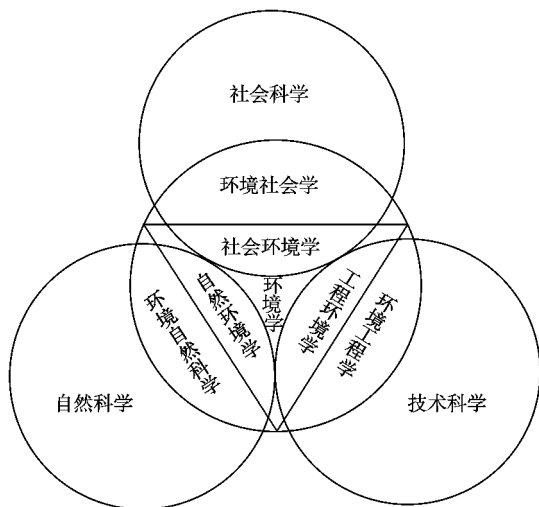
图 1-1 环境科学与相邻学科关系示意图 (据刘培同, 1988)
