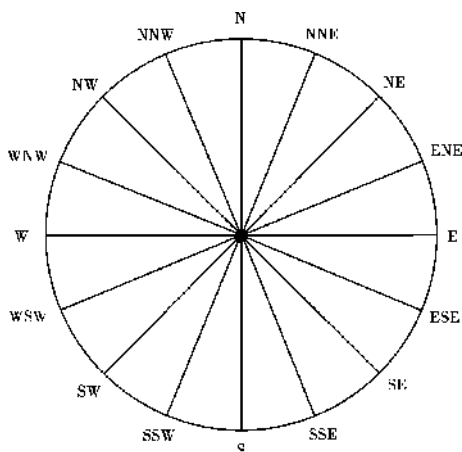
图 2.1.1 风向的方位
