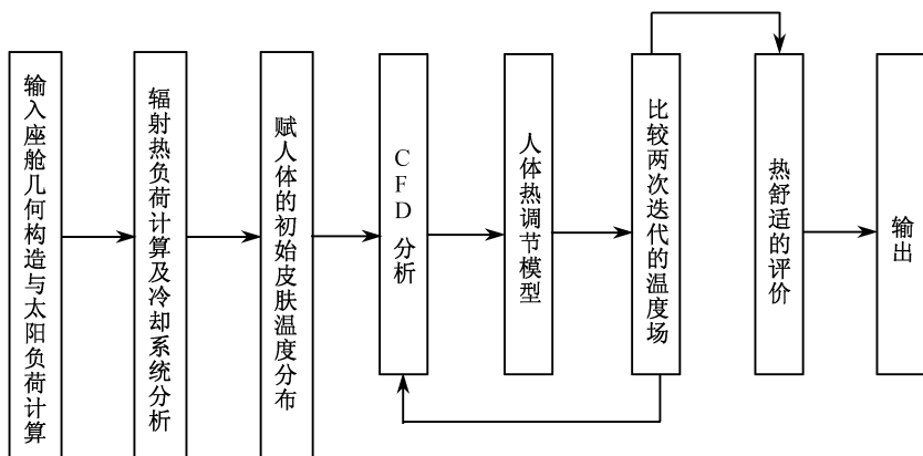
图 员摇车室内人体热舒适性的计算总框图
