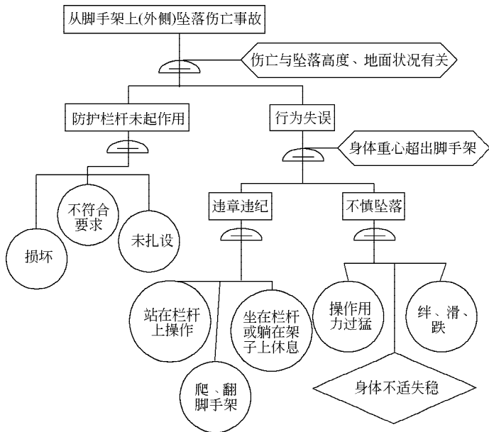
图 5-20 脚手架上坠落事故树
