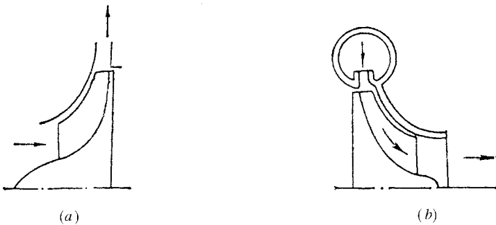
图 员原 径流式叶片机示意图 (a)离心式压气机;(b)径流式涡轮。
