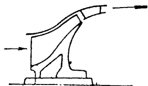
图 员原缘 斜流式压气机示意图
