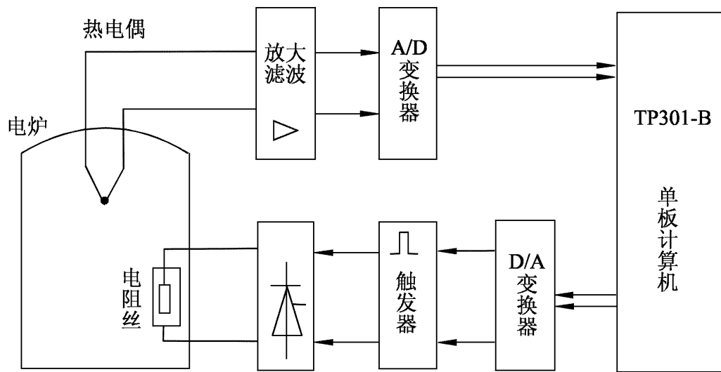
图 1-12 电阻炉温度微机控制系统
