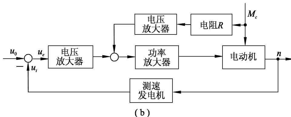
图 1-7 电动机速度复合控制系统
