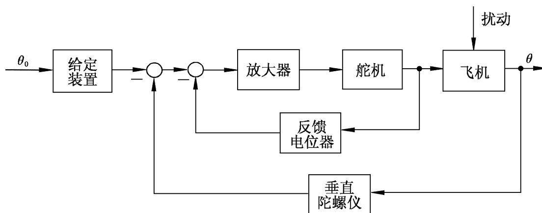
图 1-11 俯仰角控制系统方块图
