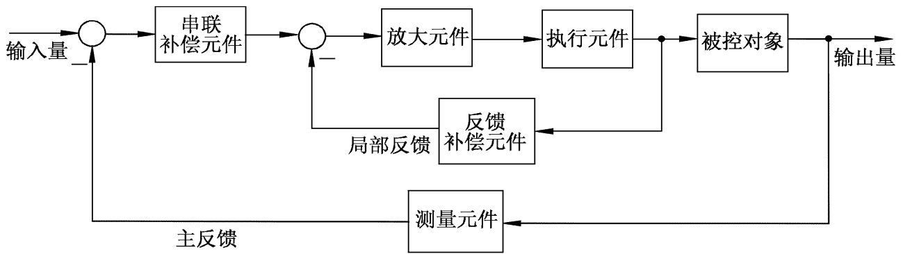
图 1-5 反馈控制系统基本组成
