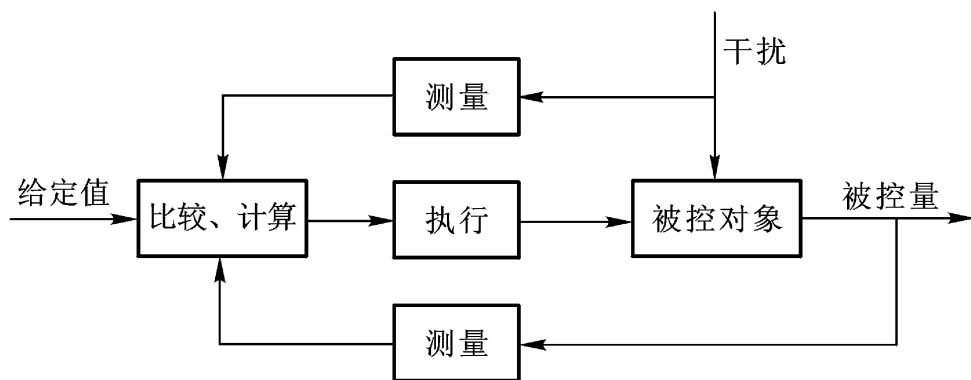
图 1 - 2 自动控制方框图
