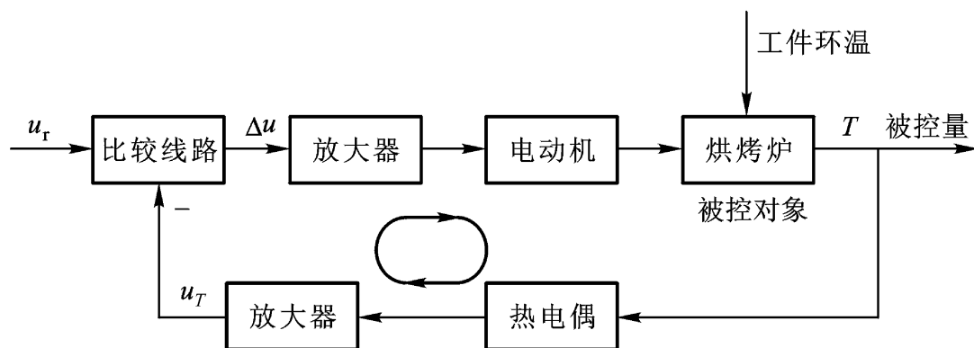
图 1 - 11 烘烤炉温度控制系统原理方框图
