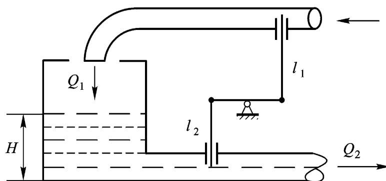
图 1 - 7 水位高度控制系统的原理图
