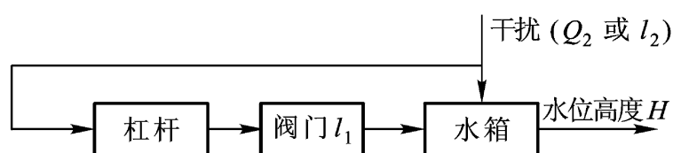
图 1 - 8 水位高度控制系统的原理方框图
