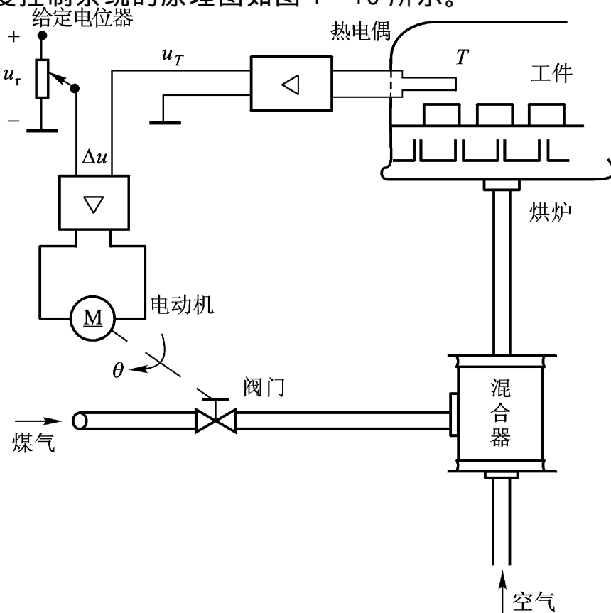
图 1 - 10 烘烤炉温度控制系统的原理图
