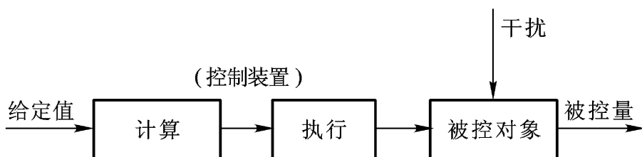
图 1 - 3 按给定值操纵的系统原理方框图
