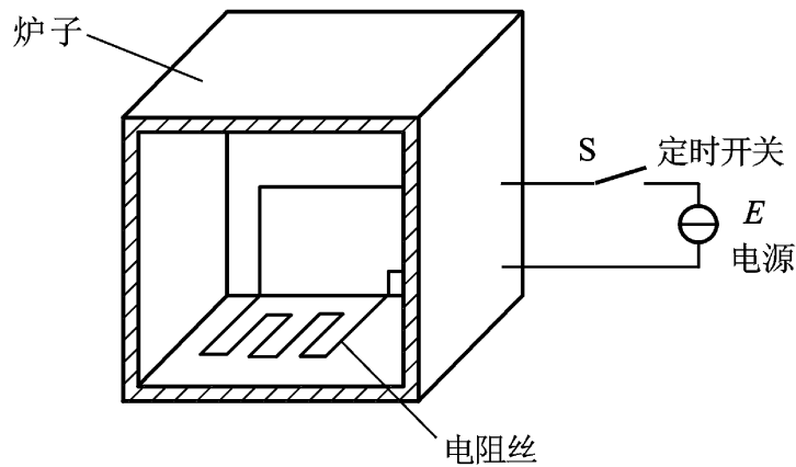
图 1 - 4 炉温控制系统的原理图
