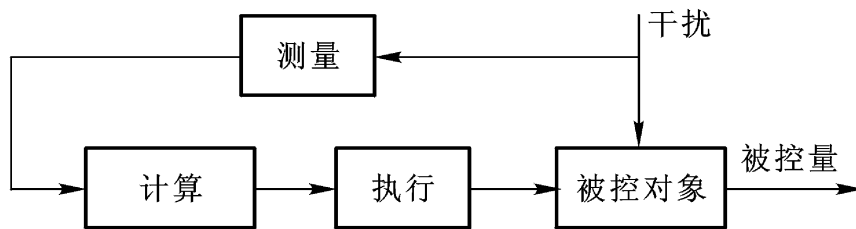
图 1 - 6 按干扰补偿的系统原理方框图
