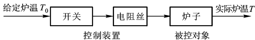
图 1 - 5 炉温控制系统的原理方框图
