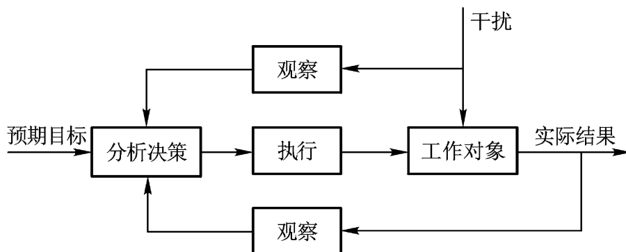
图 1 - 1 人工智能图
