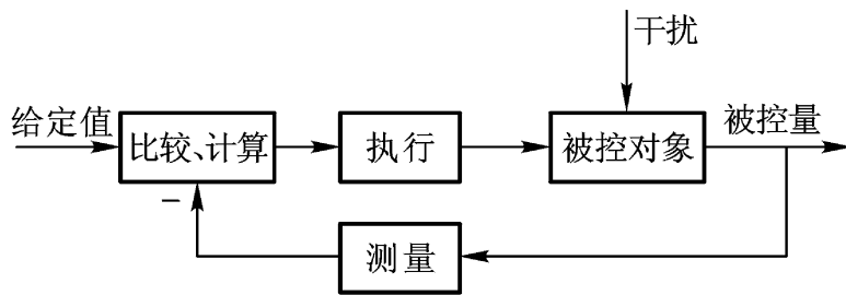
图 1 - 9 按偏差调节的系统原理方框图
