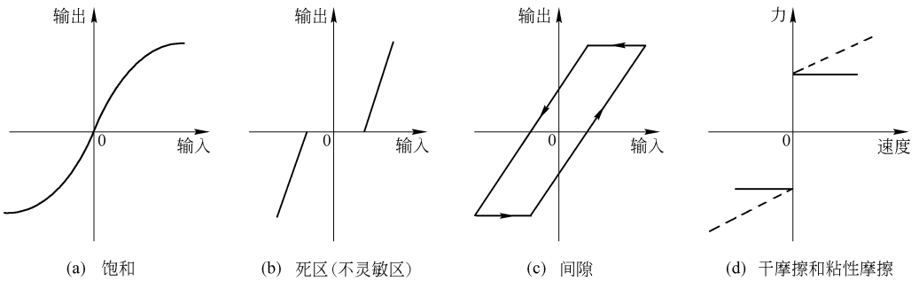
图 1-7 常见的非线性特性
