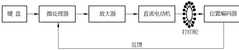
图 1.2.2 打印轮控制系统框图
