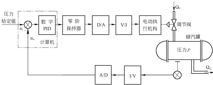
图 1.5.3 蒸汽压力闭环控制框图
