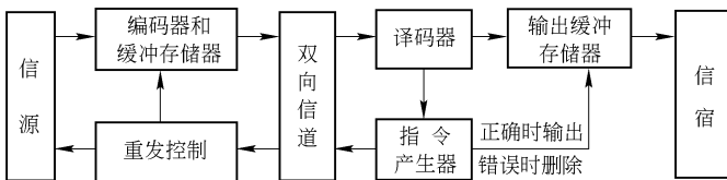
图 11.5.5 ARQ 纠错系统组成方框图
