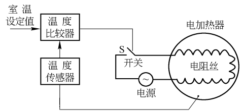
图 1.2.2 采用电加热器控制室温(闭环)示意图
