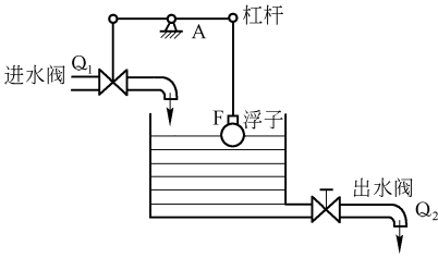
图 1.5.1 水箱示意图
