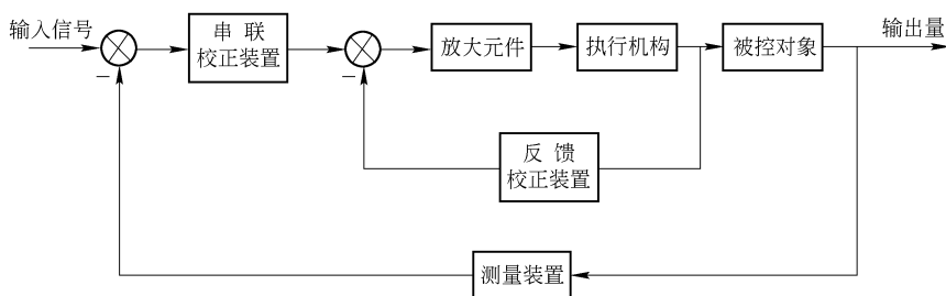
图 1-1 典型的自动控制系统方框图
