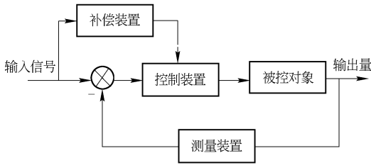
(a) 按输入作用补偿
