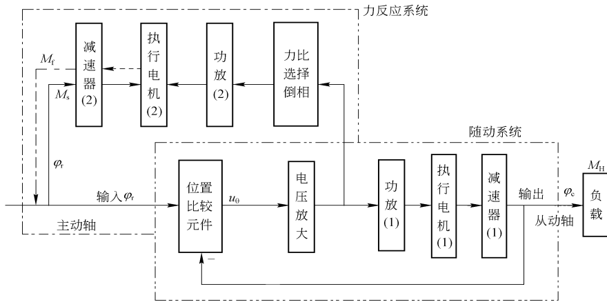
图 1.5.2 双向力反应系统结构图
