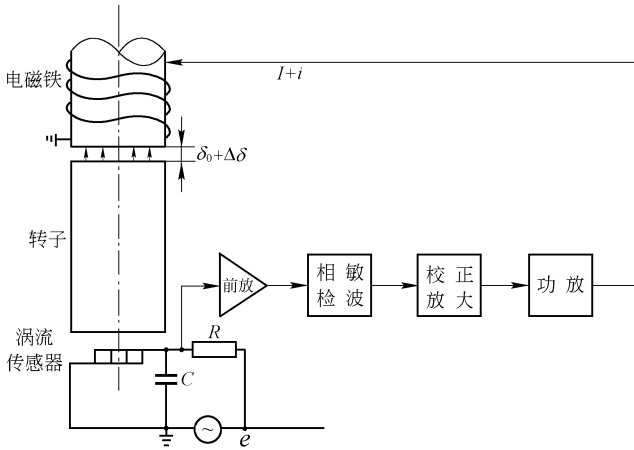
图 11.5.4 单轴磁悬浮轴承控制系统原理图
