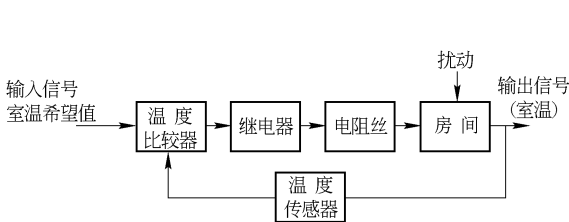
图 1.2.2 采用电加热器控制室温(闭环)示意框图
