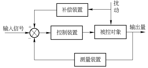
(b) 按扰动作用补偿
