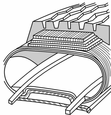
图 1-10 椭圆形载重缠绕子午线轮胎剖面
