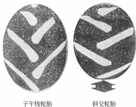
图 1-1 摇子午胎与斜交胎接地面积对比
