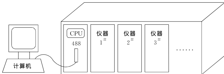
图 1-3 典型 VXI 总线仪器系统
