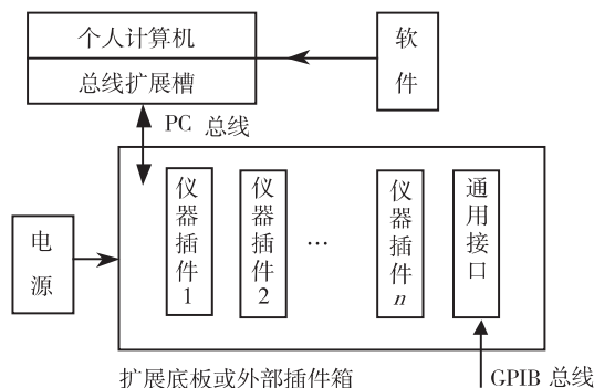
图 1-1 个人计算机仪器结构图
