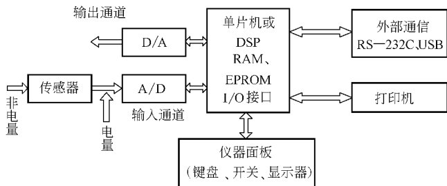
图 1-1 微机内嵌式智能仪器的基本结构
