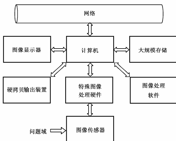
图 1-1 通用的数字图像处理系统框图
