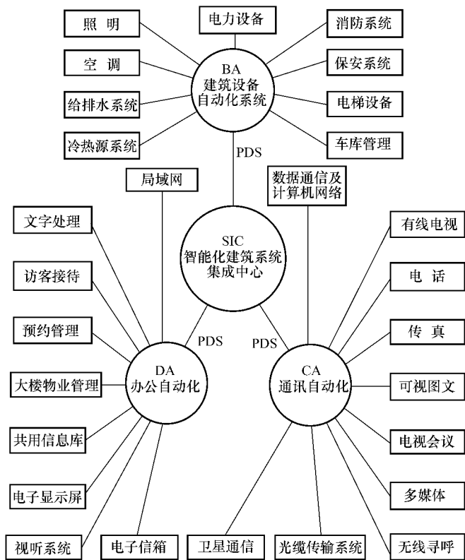
图 1-2 智能化建筑总体功能示意图
