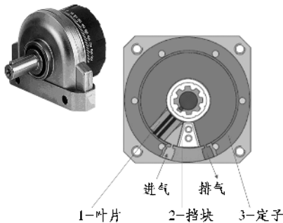
图 1-8 叶片时摆动缸
