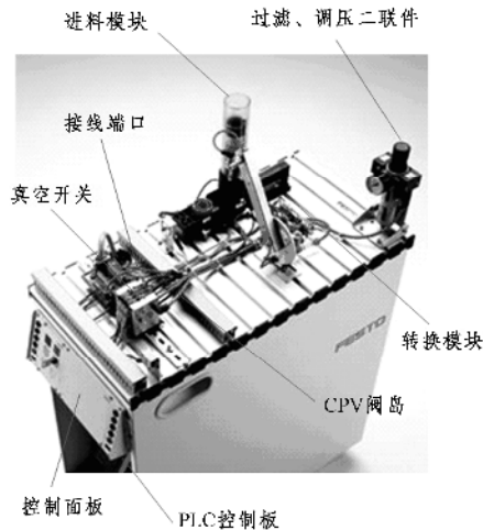
图 1-4 进料单元
