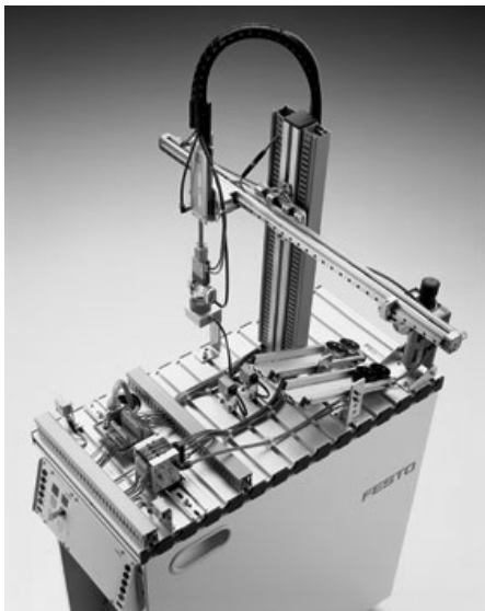
图 1-31 操作手单元
