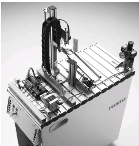
图 1-12 检测单元
