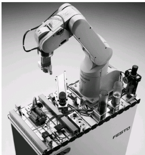
图 1-30 机械手单元
