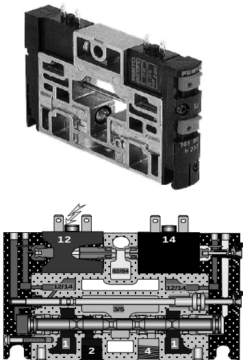
图 1-9 CPV 阀岛
