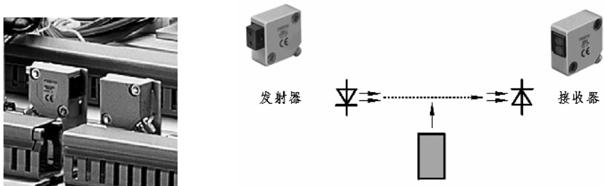
图 1-3 对射式传感器
