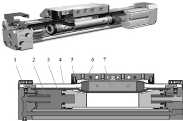
图 1-32 无杆气缸示意图
