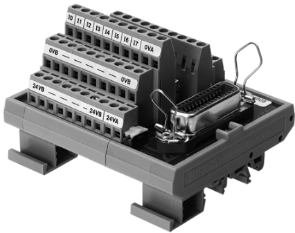
图 1-11 SYSLINK 接口
