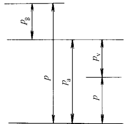
图 1-2 绝对压力、表压力、真空度之间的关系
