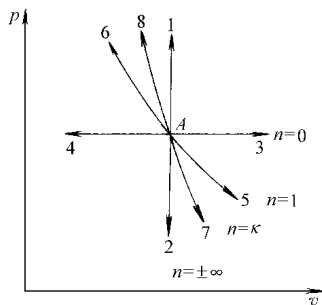
图 1-3 气体在 p - v 图上各热力过程的表示
