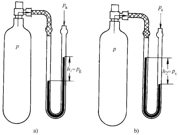
图 1-1 用液柱高度表示容器中压力值
