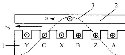
图 员原员 直线电机的基本工作原理
