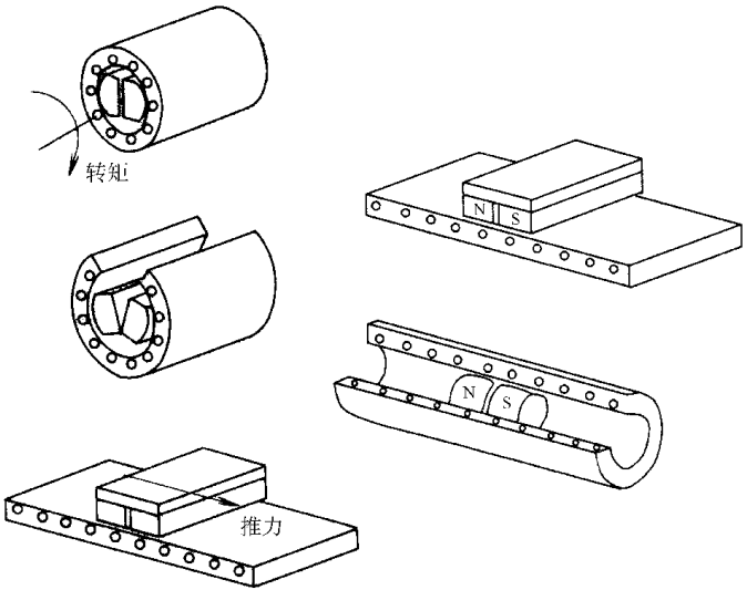
图 1-11 由永磁旋转电机演变为直线电机的过程
