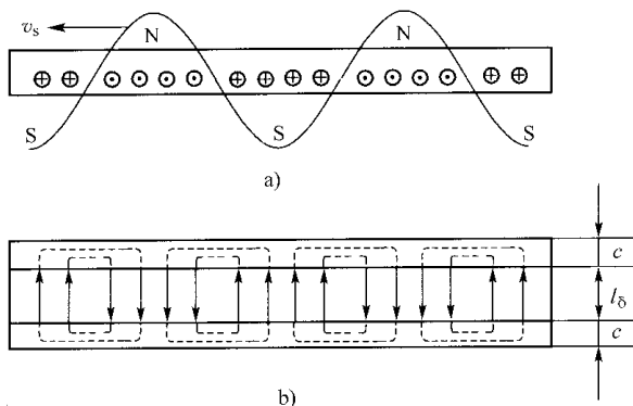
图 员原圆 次级导体板中的电流
