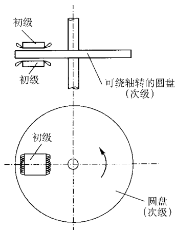
图 1-1-31 圆盘型直线电机
