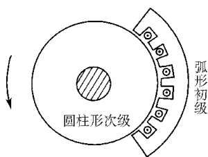
图 1-1-30 弧型直线电动机
