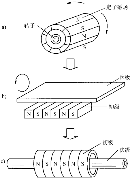
图 15-10 旋转电机演变为圆筒型直线电机的过程 1) 旋转电机 2) 扁平型单边直线电机 3) 圆筒型(管型)直线电机
