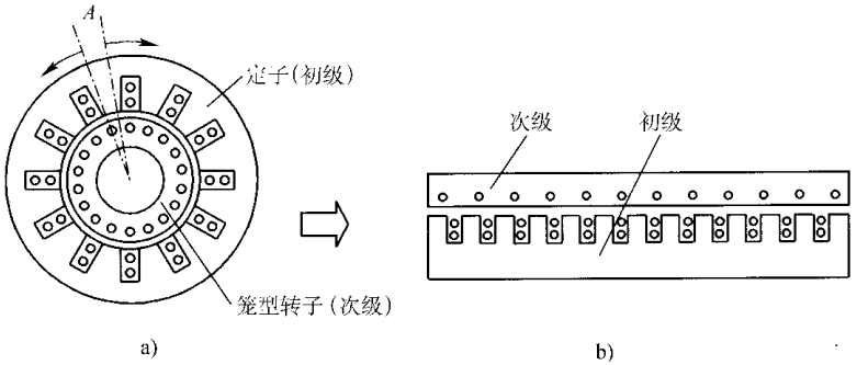
图 1-10 由感应式旋转电机演变为直线电机的过程
