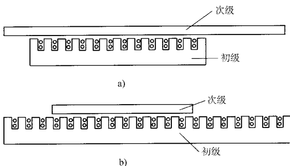
图 1 单边型直线电机
