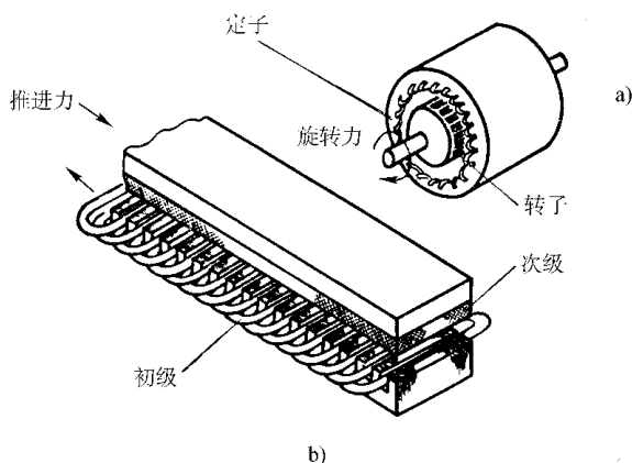
图 猿圆猿 旋转电动机和直线电动机示意图
