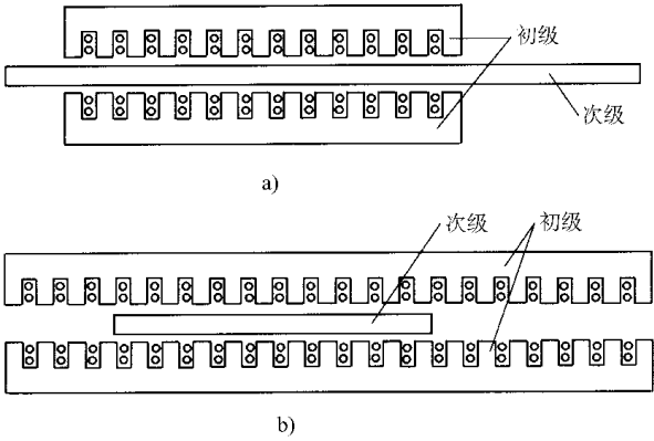
图 15-9 双边型直线电机 1) 短初级 2) 短次级
