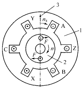
图 员原园 旋转电机的基本工作原理
