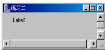
图 2-3 出现滚动条
