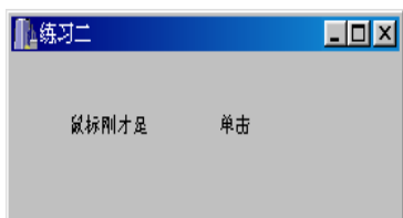
图 2-8 事件响应
