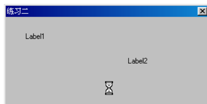
图 2-5 对话框格式
