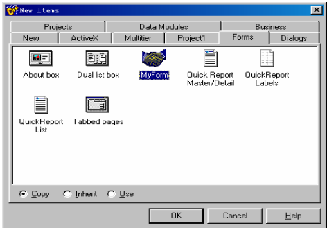
图 2-10 自己的模板
