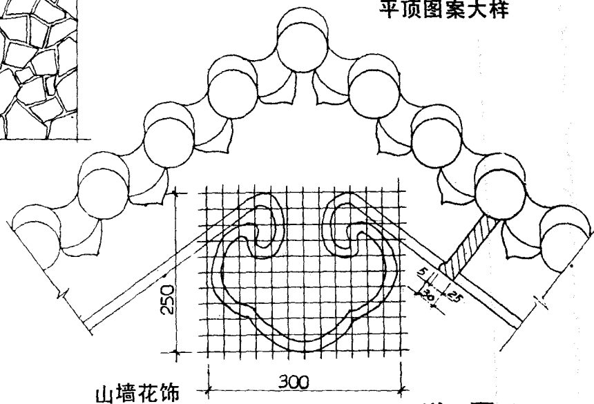
(4) 详图(四)
