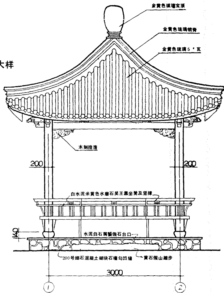
立面图
