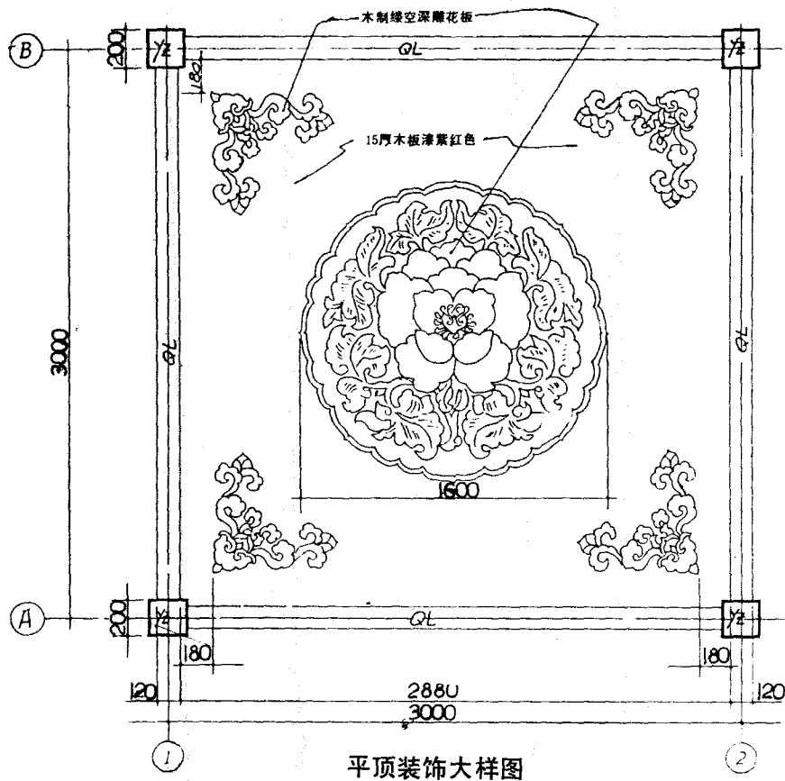
木制镂空花板挂落大样
