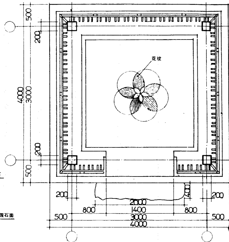
平面图
