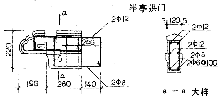
YYD配筋图
