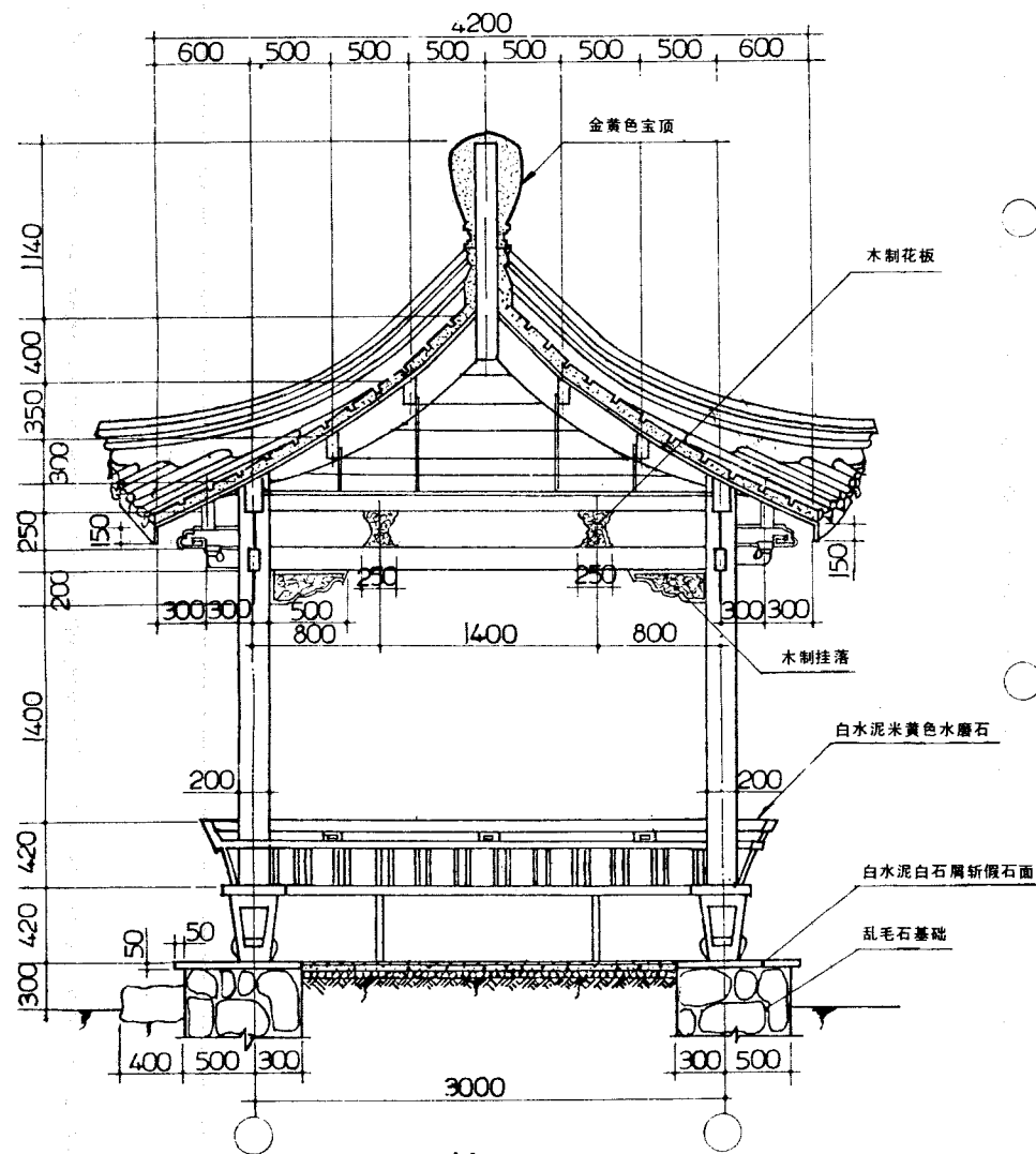
剖面图
